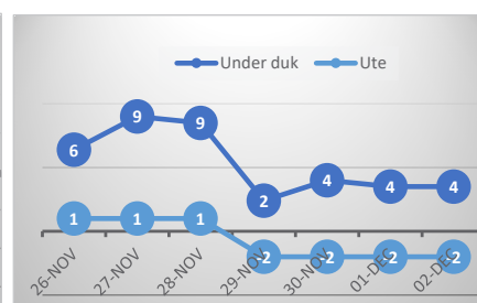
Bild 6. Hämtat från en odlarintervju: Utomhustemperatur resp. temperatur under fiberduk i ett tunnelväxthus för lägsta och högsta dygnstemperatur. T.v Lägsta nattetemperatur 26 nov – 2 dec 2014. T.h Högsta dagstemperatur 26 nov – 2 dec 2014. Odlarkommentar: trots att vi ibland har ner till -20 grader ute så går temperaturen sällan under -5 grader under fiberduken i tunneln.
