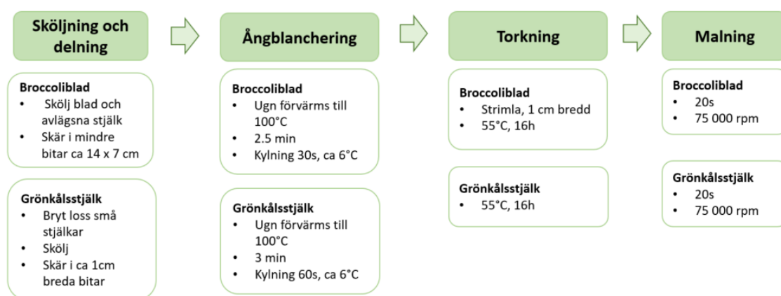
Figur 4. Metodik för framställning av pulver av brocoliblad och grönkålsstjälk.
